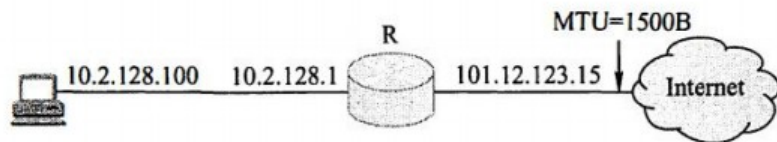
题 47-a 图 网络拓扑
